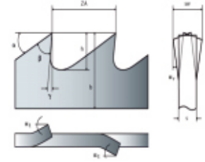
Band saw blade tip angle Şerit testere bıçağı uç açısı
